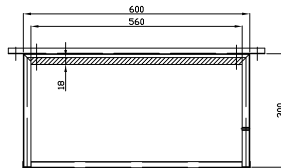
DOORSNEDE B-B
